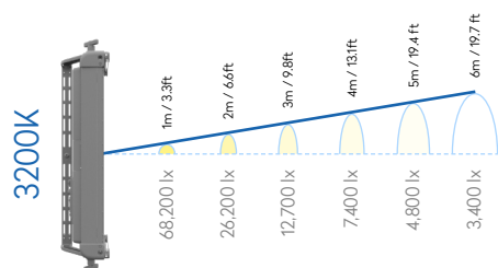
いすなし標準ビーム角20°
